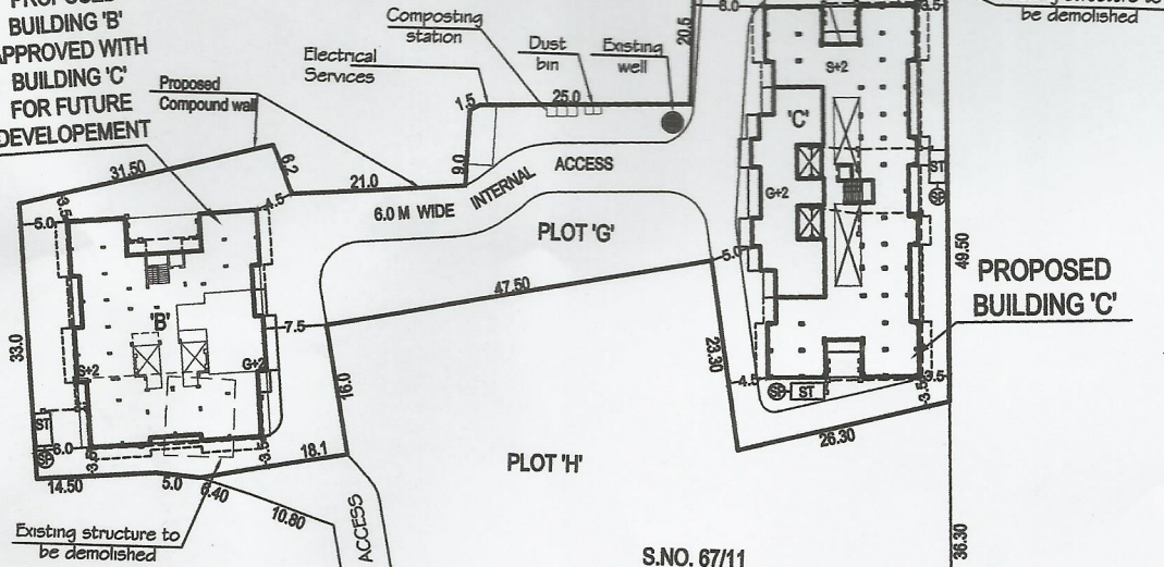
SITE PLAN 1:1000
