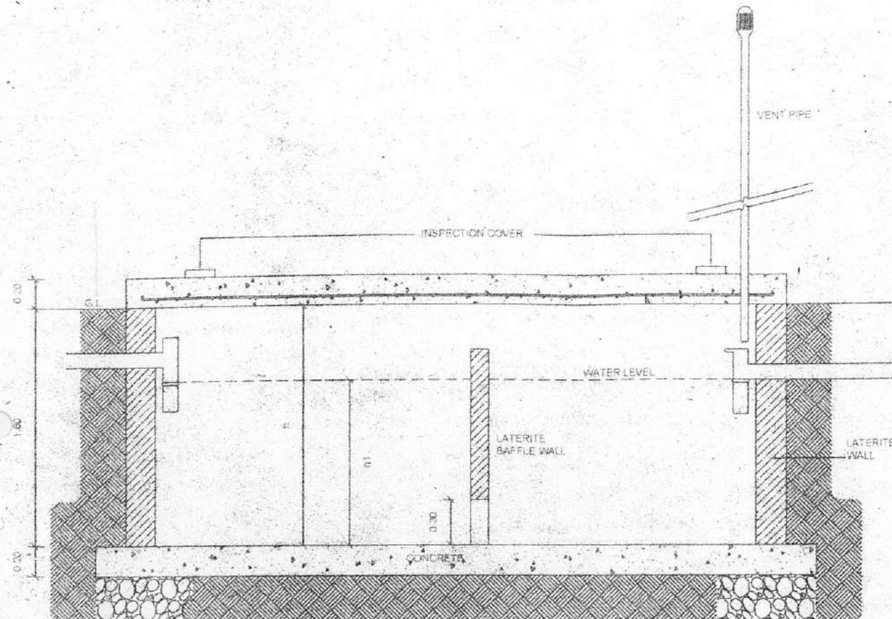
LONGITUDINAL SECTION
