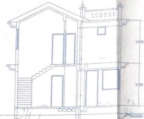
SECTION A-A SC 110
