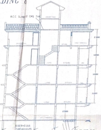
SECTION A-A SC. 1:100
