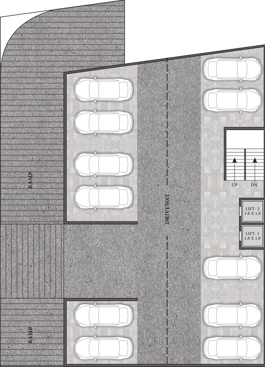
U. BASEMENT FLOOR
